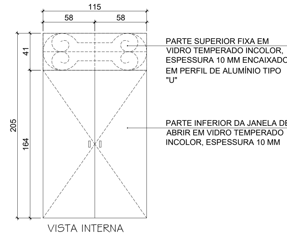
J1 - 115 X 205 CM (X4) ESC: 1/25
