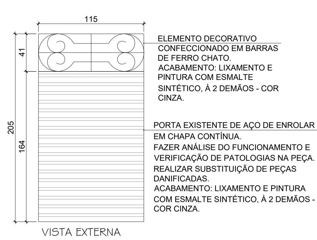
J1 - 115 X 205 CM (X4) ESC: 1/25
