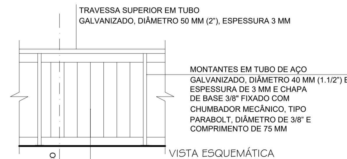
GRADIL FORMADO POR BARRA CHATA, AÇO ASTM A 36, DIMENSÕES 1.1/2" X 3/16" (32 X 4,8 MM)
