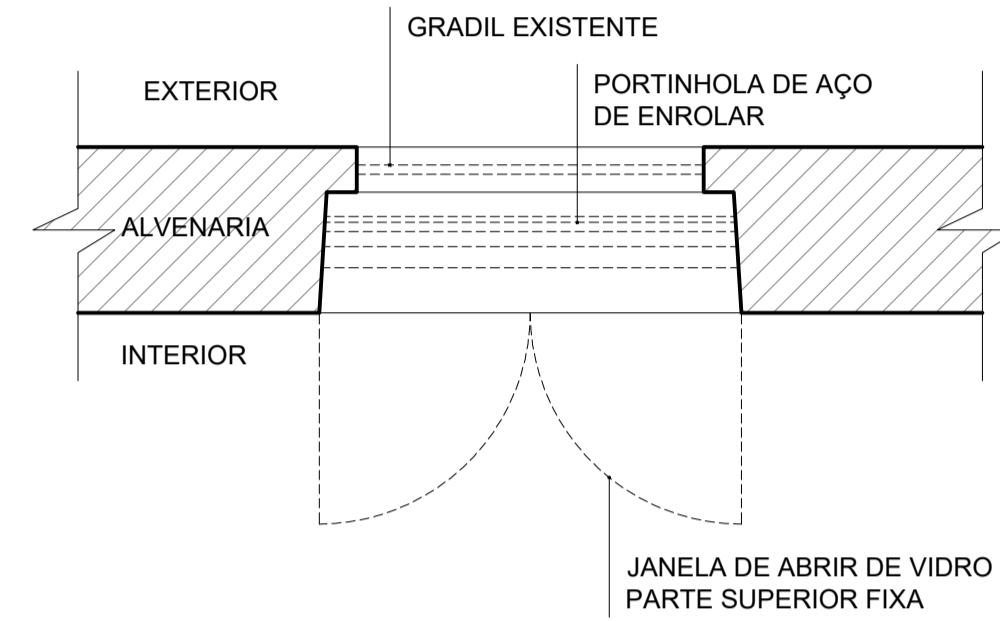
J1 - 115 X 205 CM (X4) ESC: 1/25
