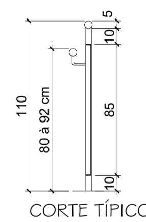
GUARDA-CORPO E CORRIMÃO ESC: 1/25 ACABAMENTO: PINTURA EM ESMALTE SINTÉTICO COR BRANCO
