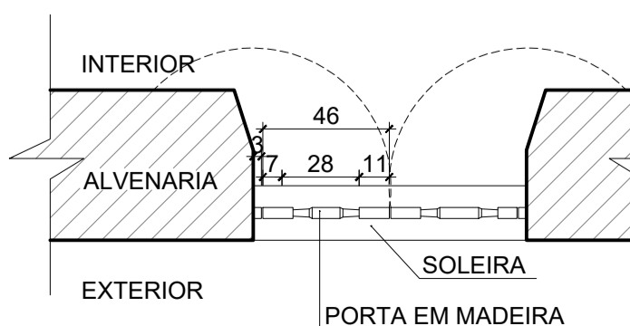
P6 - 100 X 305 CM (X1) ESC: 1/25 ACABAMENTO: EMASSAMENTO A ÓLEO E PINTURA EM ESMALTE SINTÉTICO COR CINZA CLARO.
