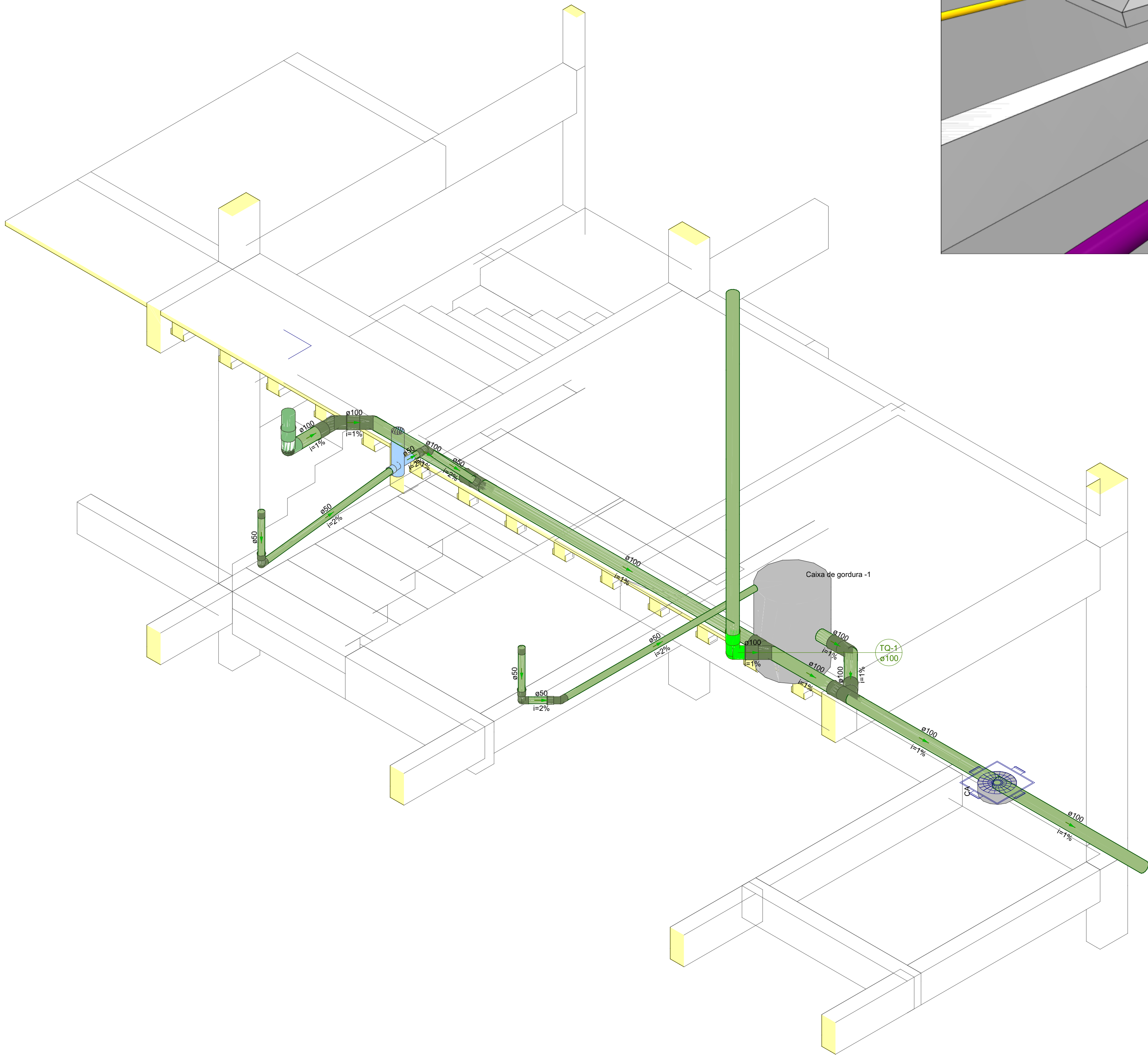
Detalhe SAN-1 Escala 1:25
