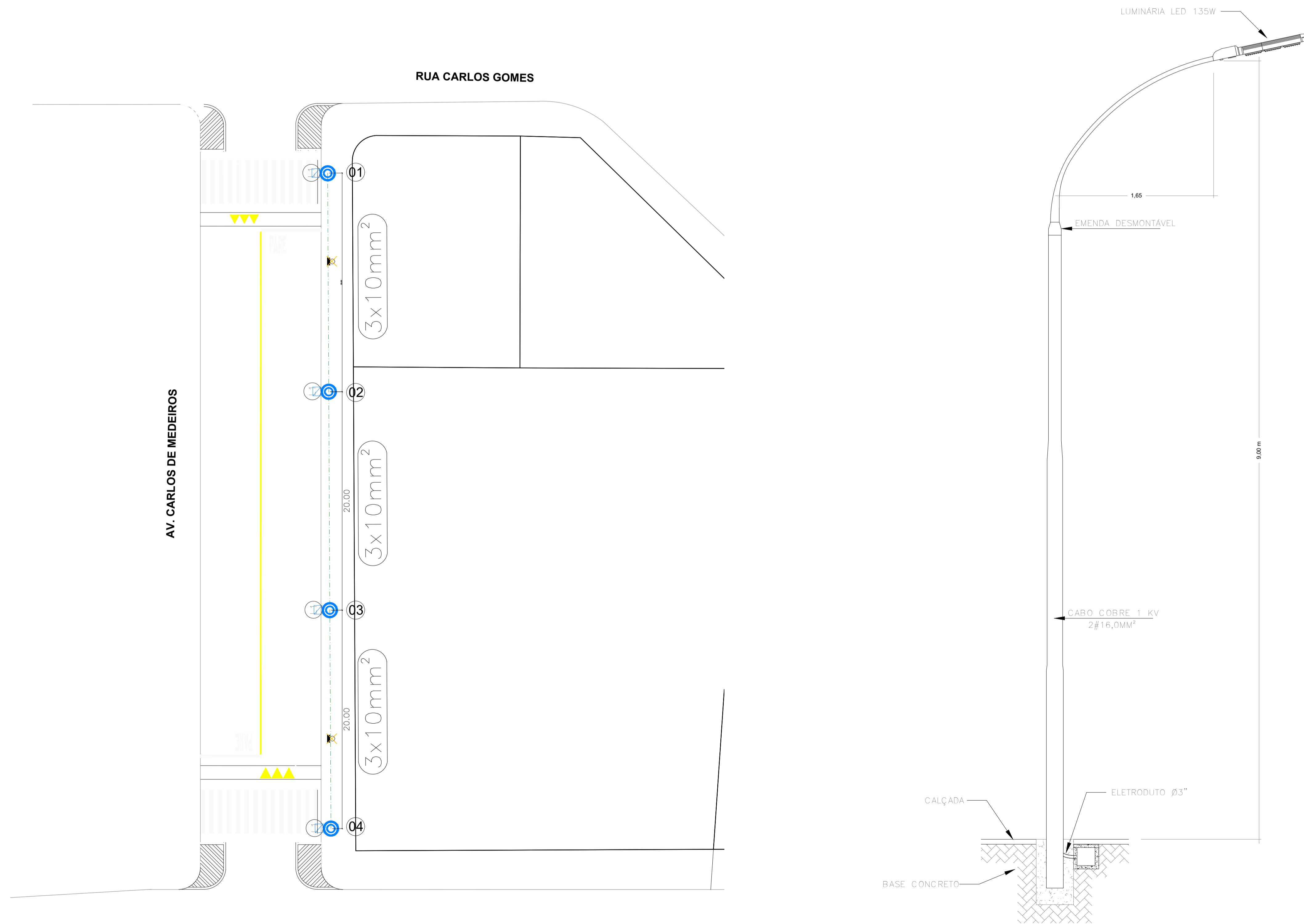
DETALHE - POSTE DE AÇO GALVANIZADO CURVO SEM ESCALA
