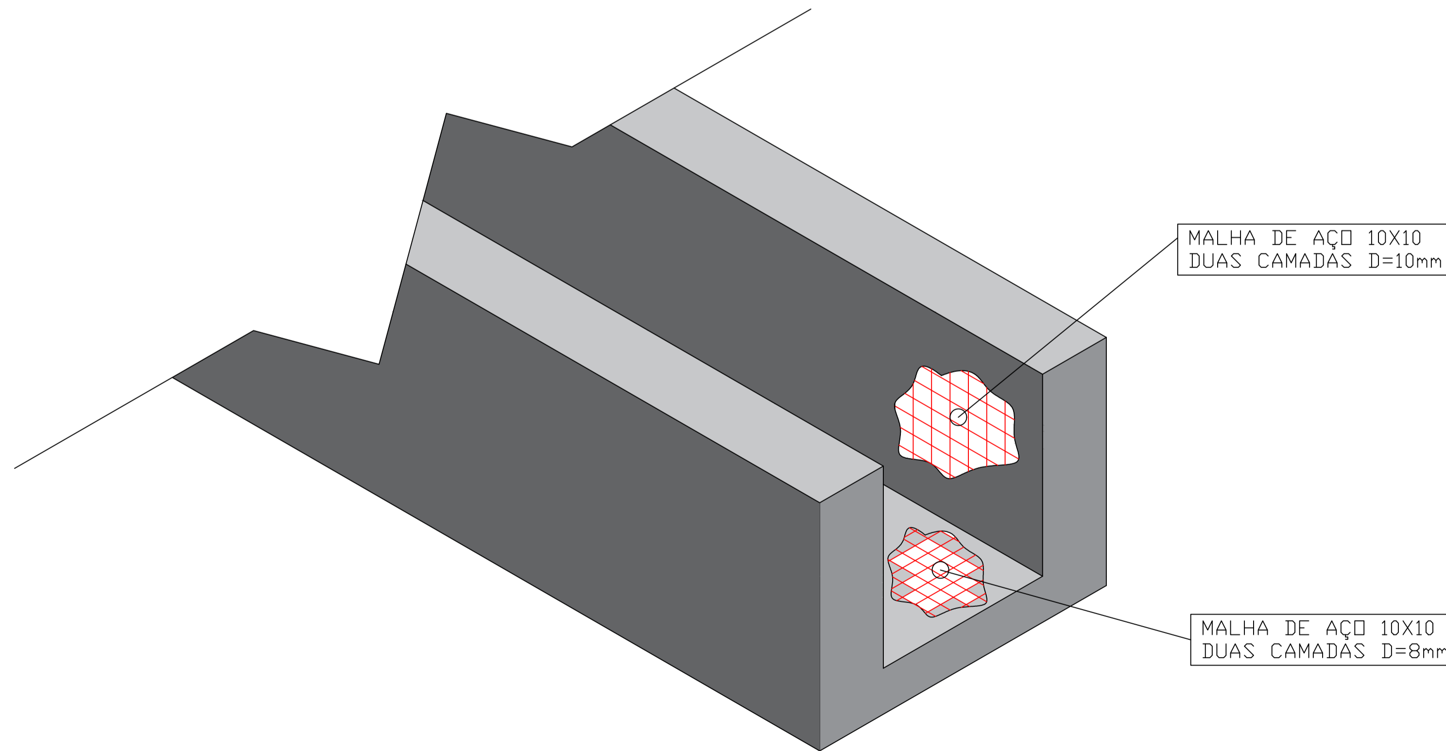
DETALHE ISOMÉTRICO ESC.: 1:20
