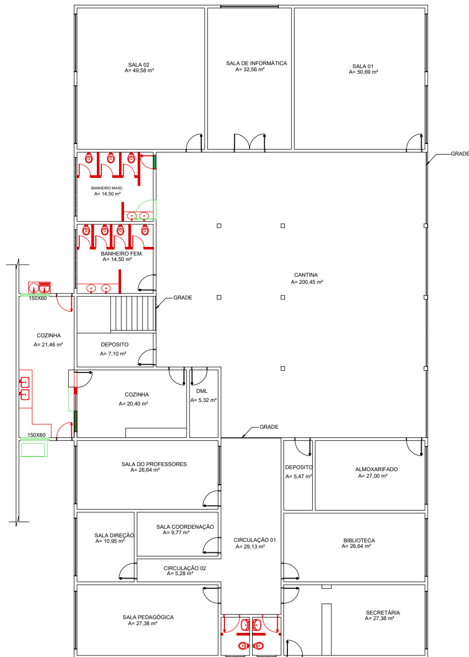
○ PLANTA BAIXA DE REFORMA – PAVIMENTO TÉRREO ESC.: 1:200
