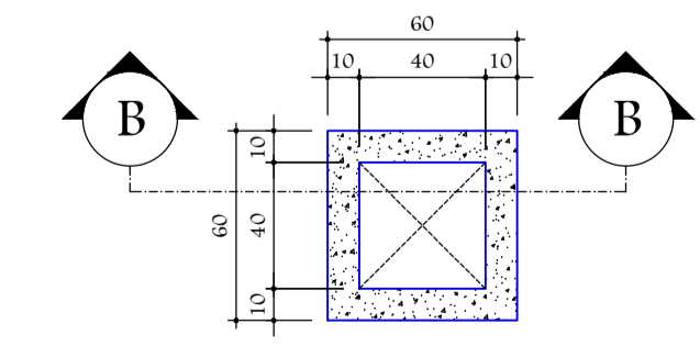
PLANTA BAIXA - CAIXA DE PASSAGEM ESCALA: 1/25
