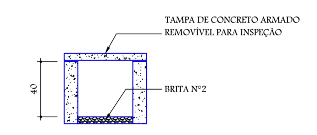
CORTE - CAIXA DE PASSAGEM ESCALA: 1/25
