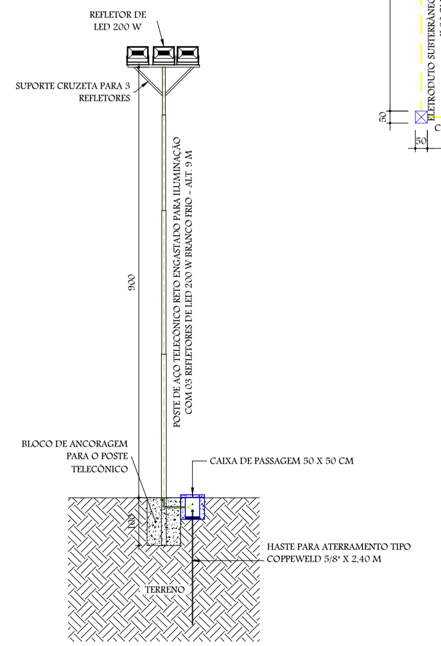
DETALHE POSTE COM REFLETORES ESCALA: 1/75
