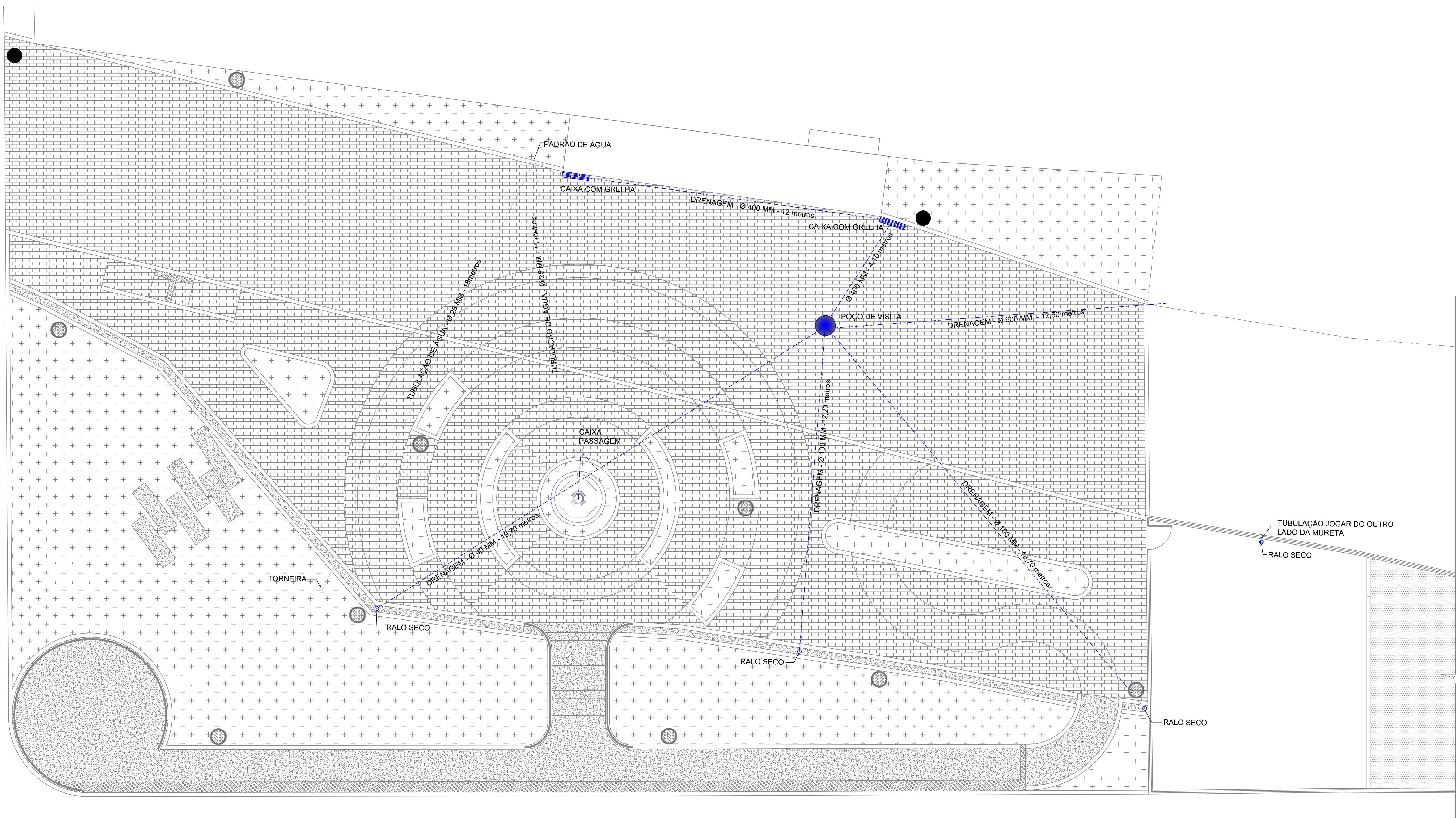
PLANTA BAIXA -- PONTOS HIDRÁULICOS E TUBULAÇÕES DE DRENAGEM ESC.: 1:75
