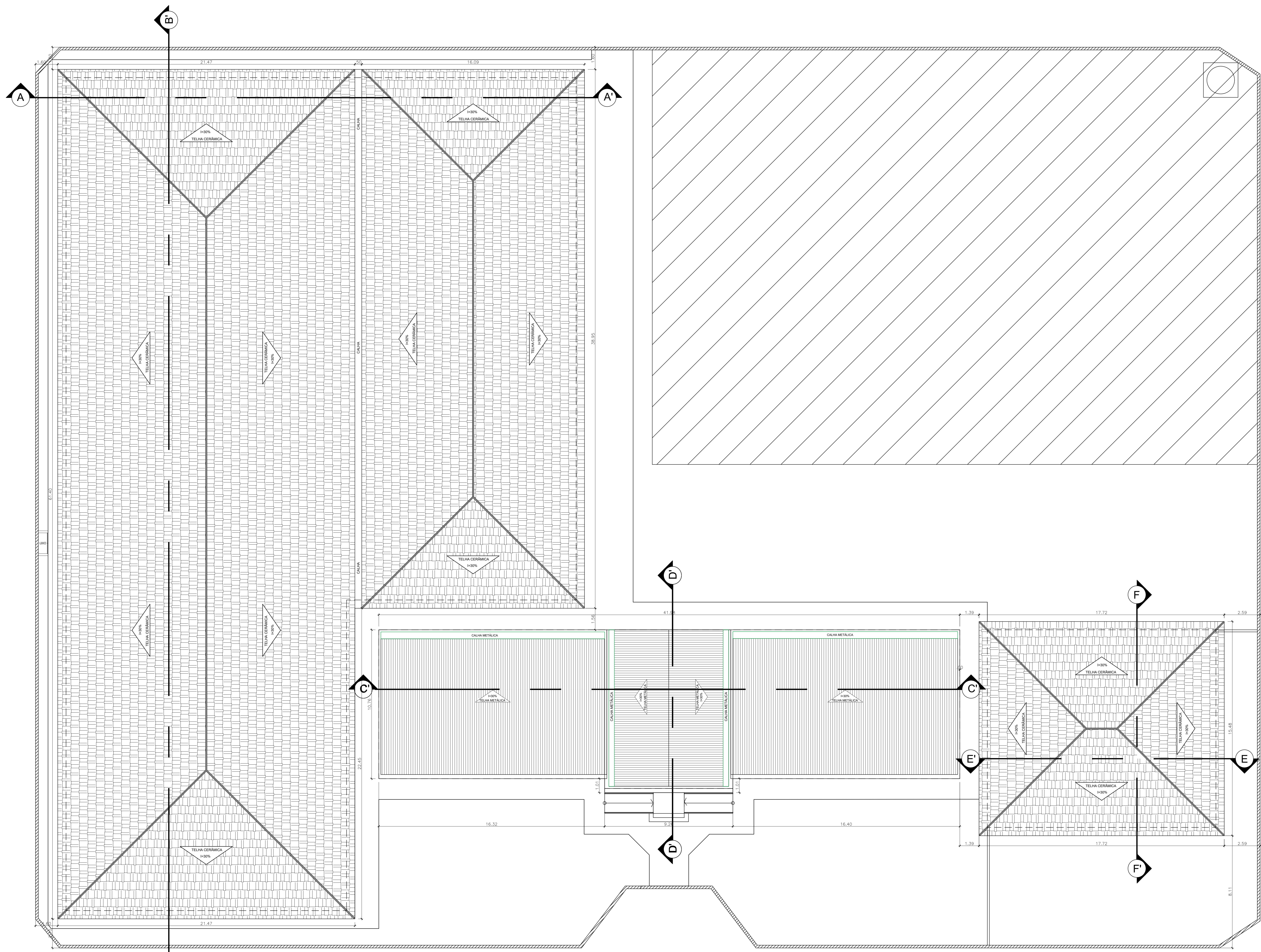
PLANTA BAIXA - TELHADO ESCALA 1/100
