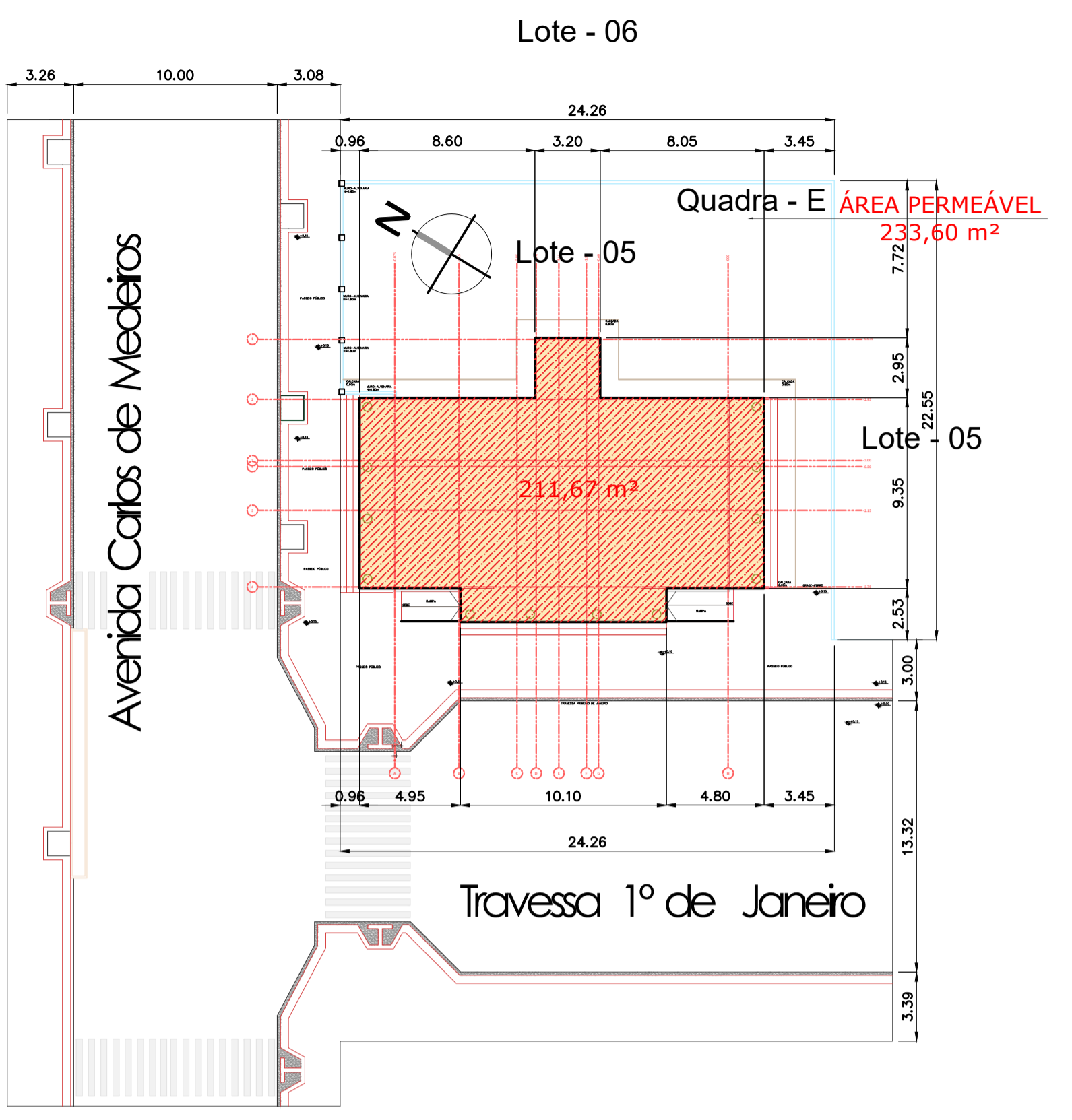
PLANTA IMPLANTAÇÃO ESC. 1:250
