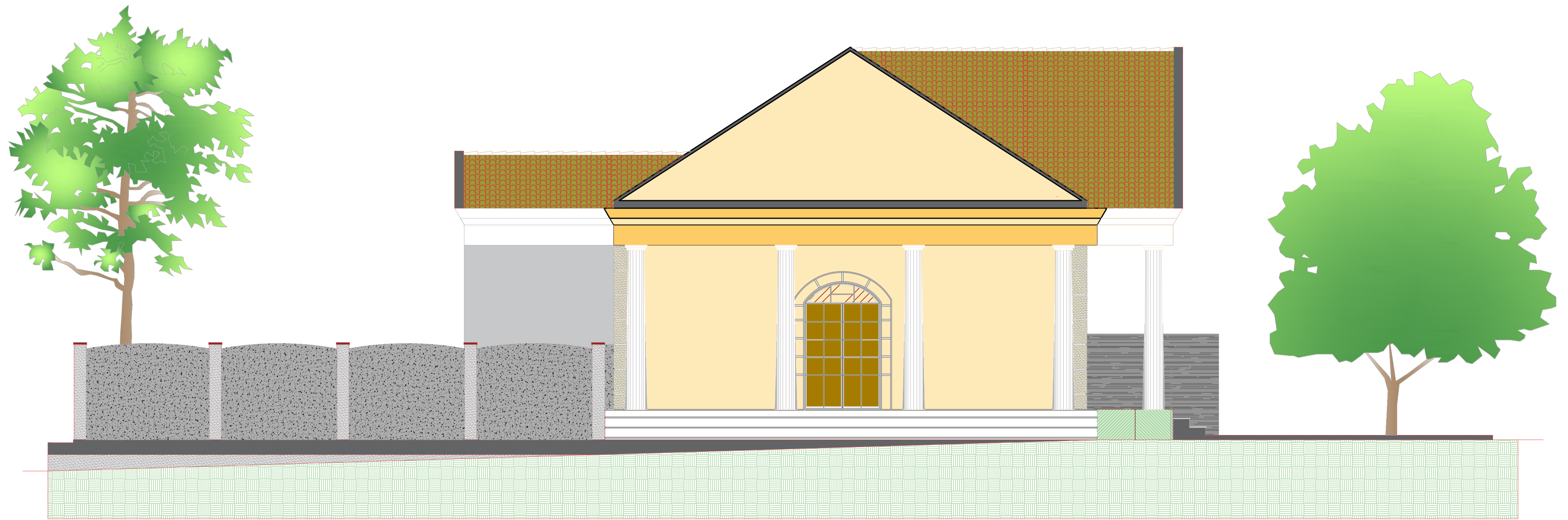
FACHADA - AVEN. CARLOS DE MEDEIROS ESC. 1:50
