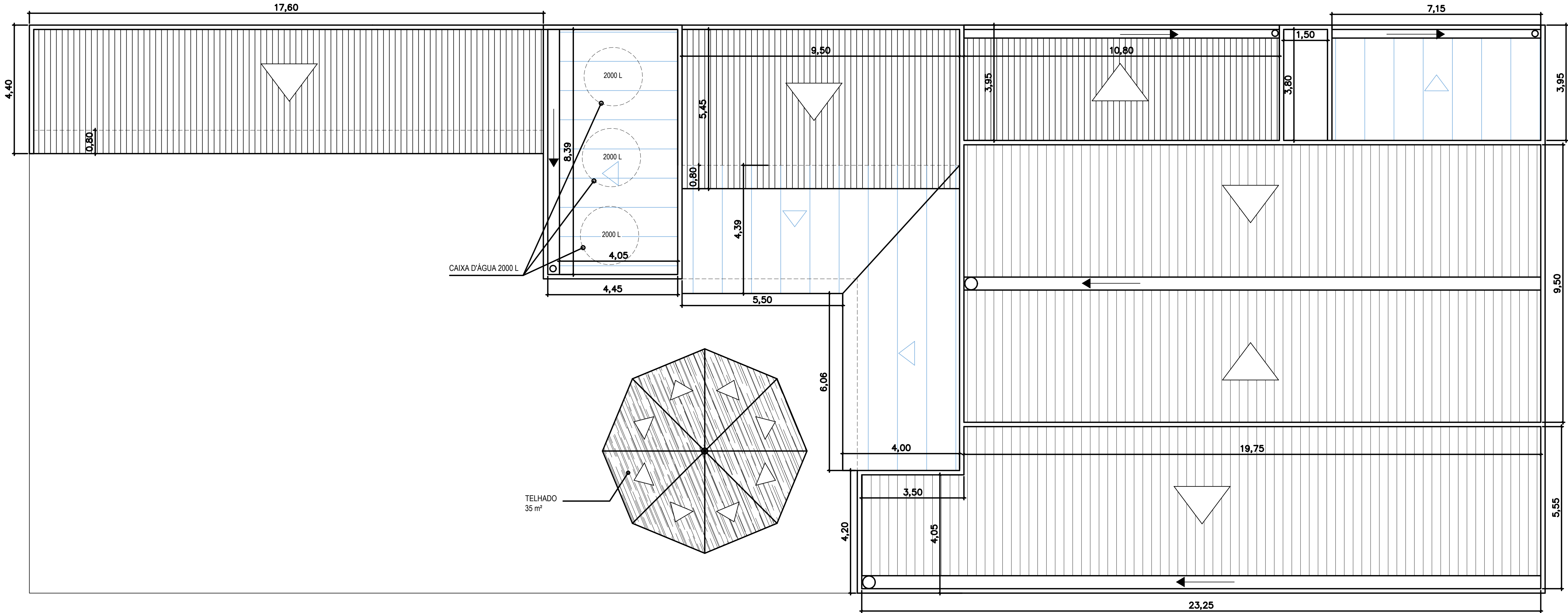
PLANTA BAIXA – COBERTURA ESCALA.: 1: 75
