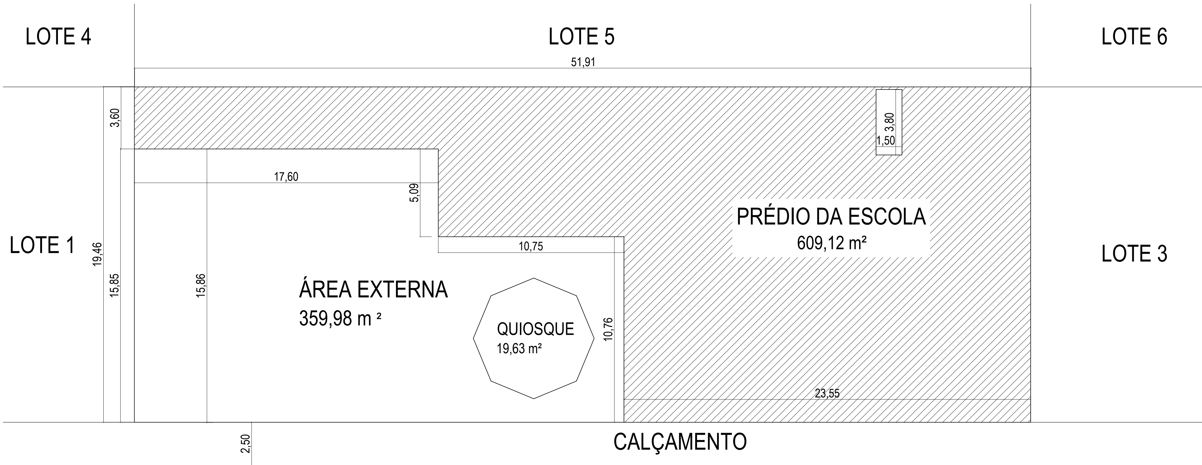
PLANTA BAIXA – COBERTURA ESCALA.: 1: 75
