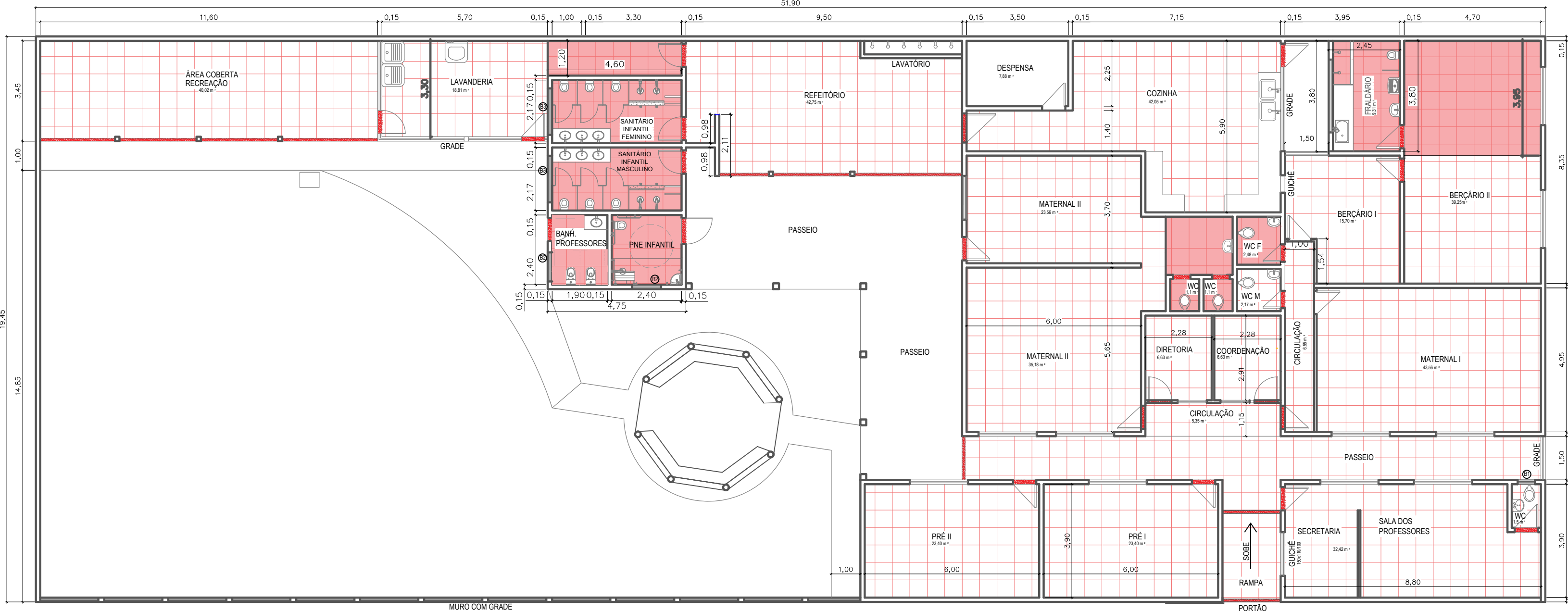
PLANTA BAIXA – REFORMA – PISOS ESCALA.: 1:125
